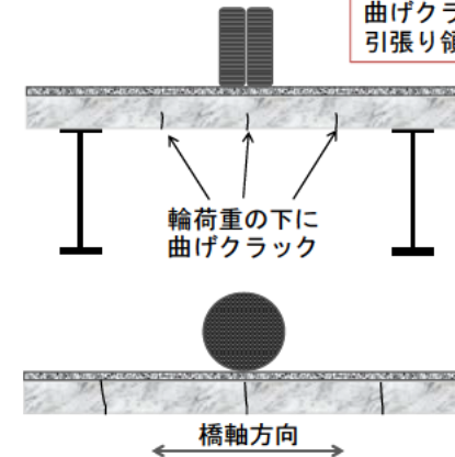
曲げクラック
