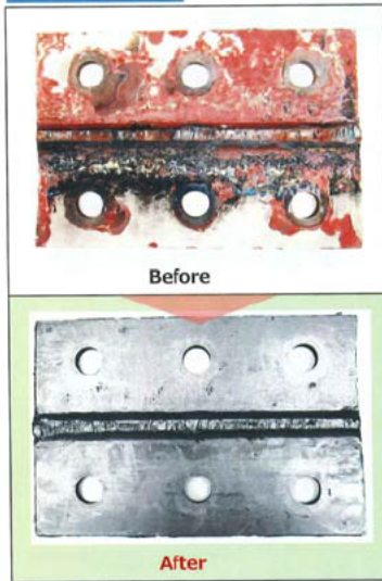
塗装、サビ除去の例
